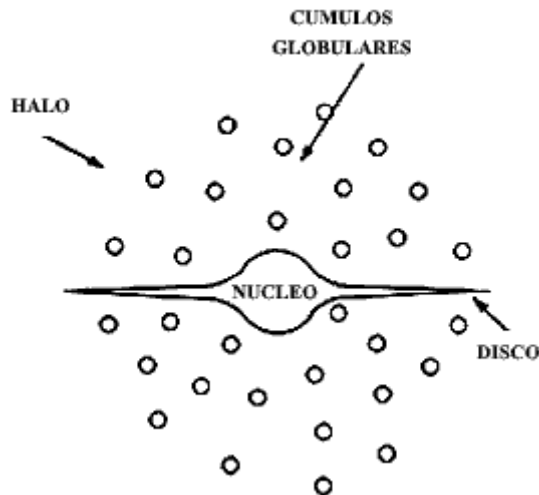
Figura 44. Esquema de una galaxia elíptica.
