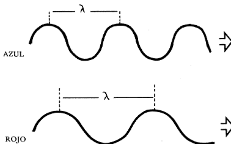
Figura 12. La luz es una onda electromagnética. La longitud de la onda \lambda . Determina el color (véase también la figura 34).
