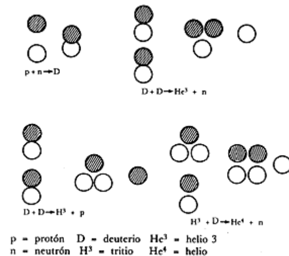
Figura 37. Producción de un núcleo de helio a partir de protones y neutrones.
