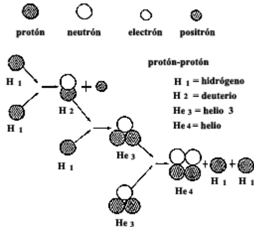
Figura 42. El ciclo protón-protón
