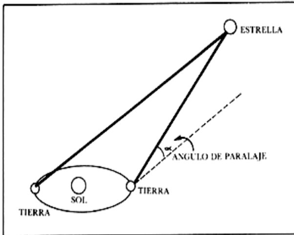
Figura 6. Midiendo el ángulo de paralaje \alpha y conociendo el radio de la órbita terrestre, se deduce la distancia a una estrella.
