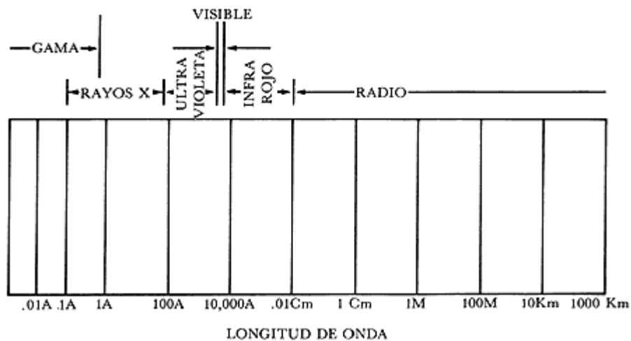
Figura 31. El espectro electromagnético. La luz corresponde a un pequeño rango de frecuencias ( \text{\AA} = Angstrom = 10^{-8} cm).
